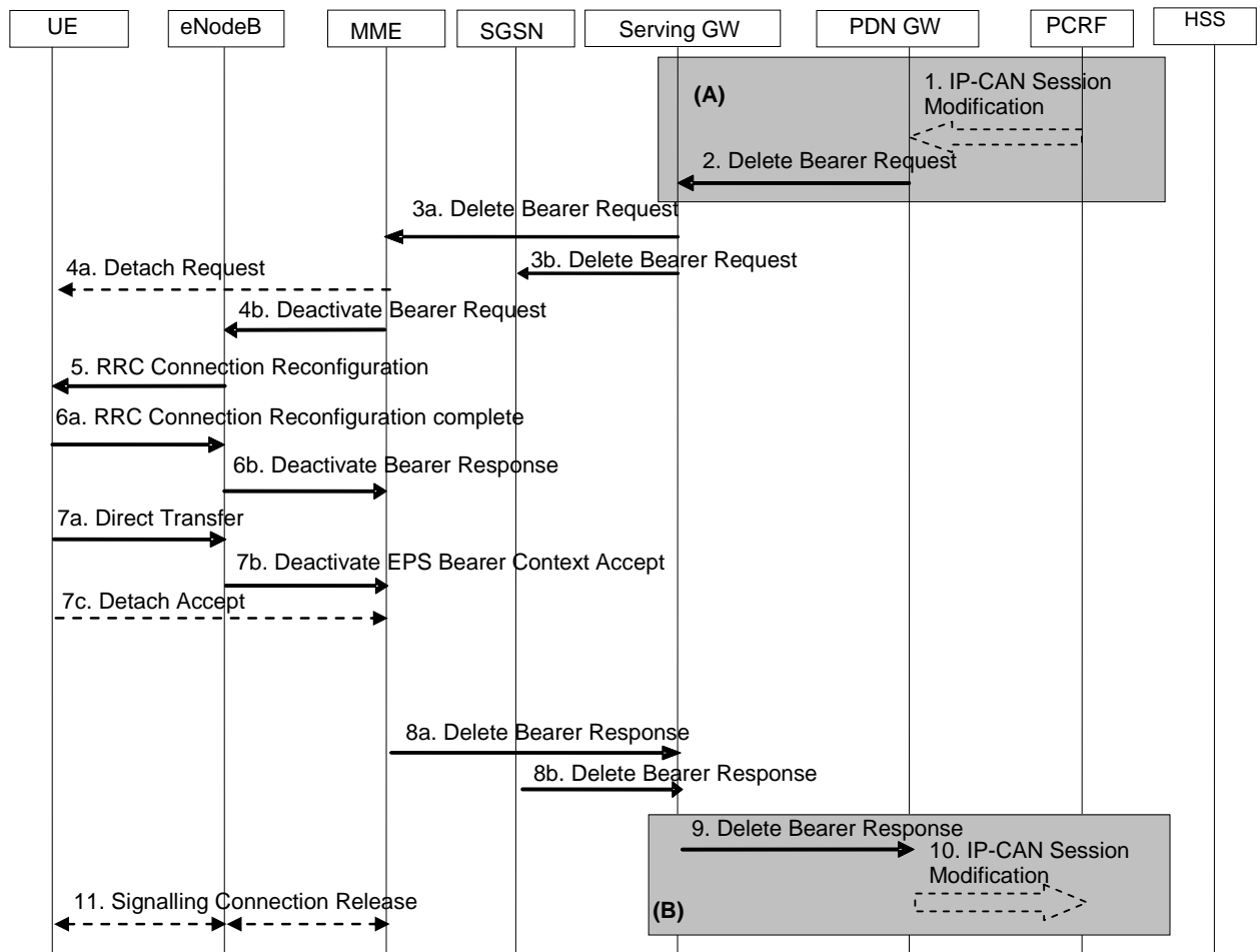
Рис.8.12. Процедура деактивации сквозного канала; UE в состоянии CONNECTED
