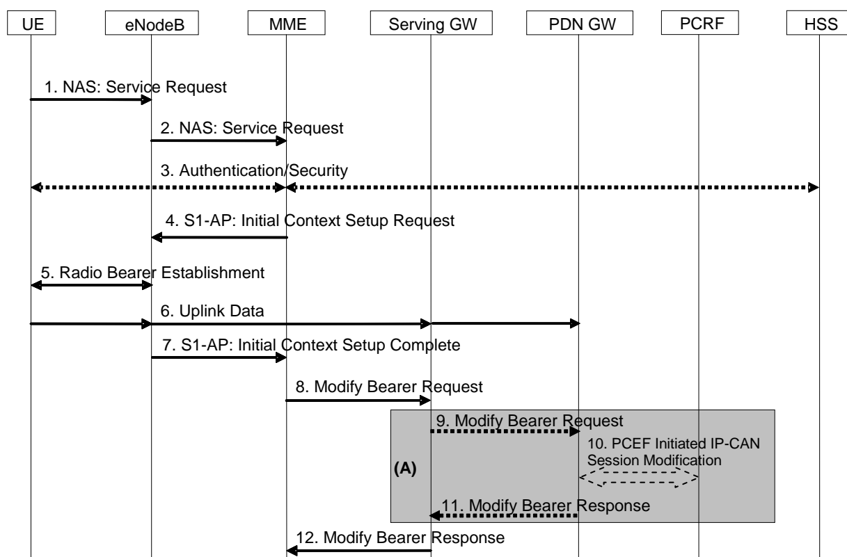
Рис.8.6. Процедура Service Request, запускаемая UE
