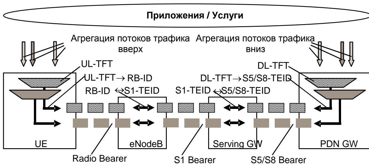
Рис.7.1. Структура двух сквозных каналов
