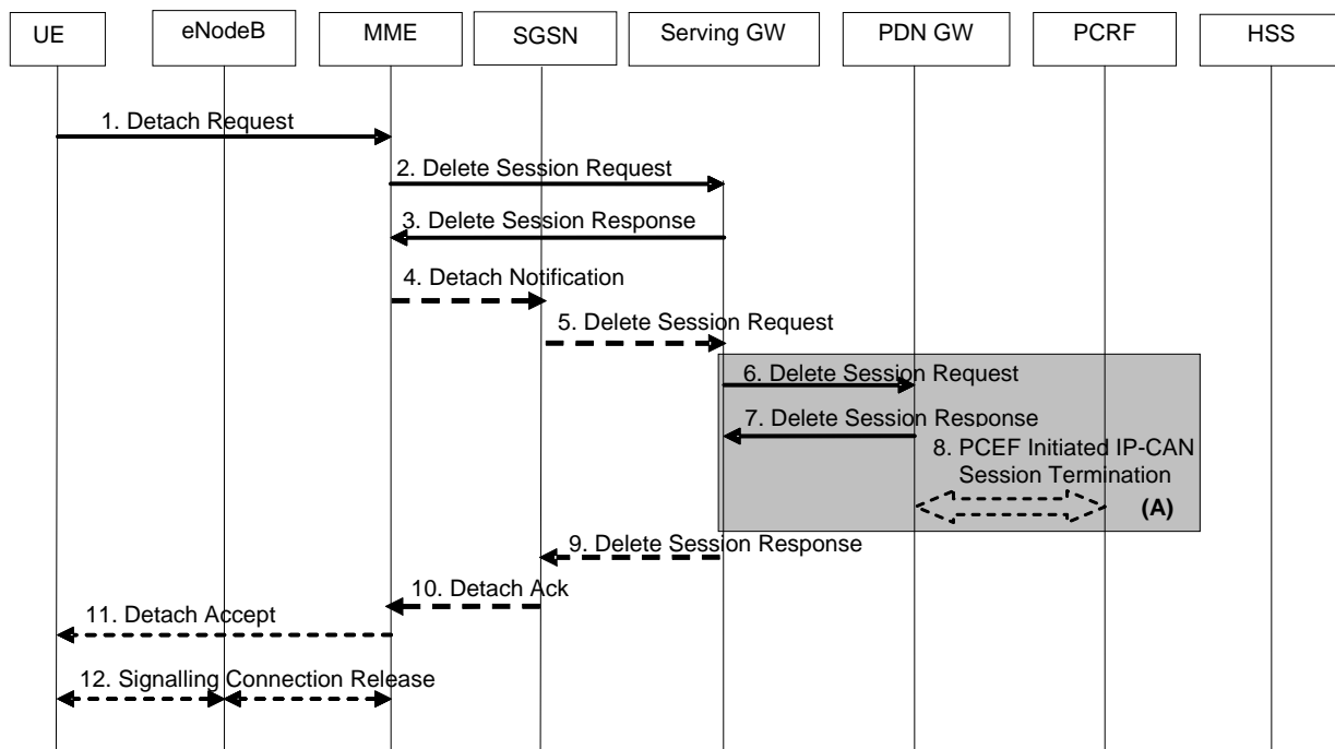
Рис.8.8. Процедура Detach
